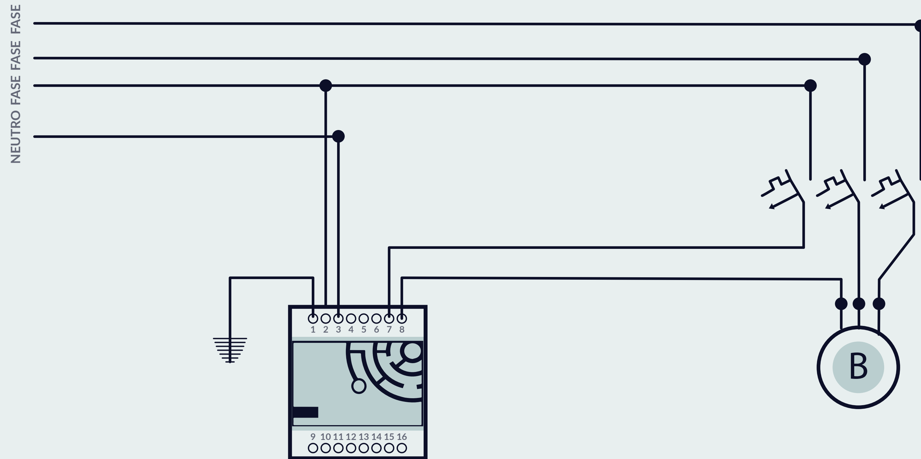
Figura 1: Esquema unifilar de conexión bomba monofásica
