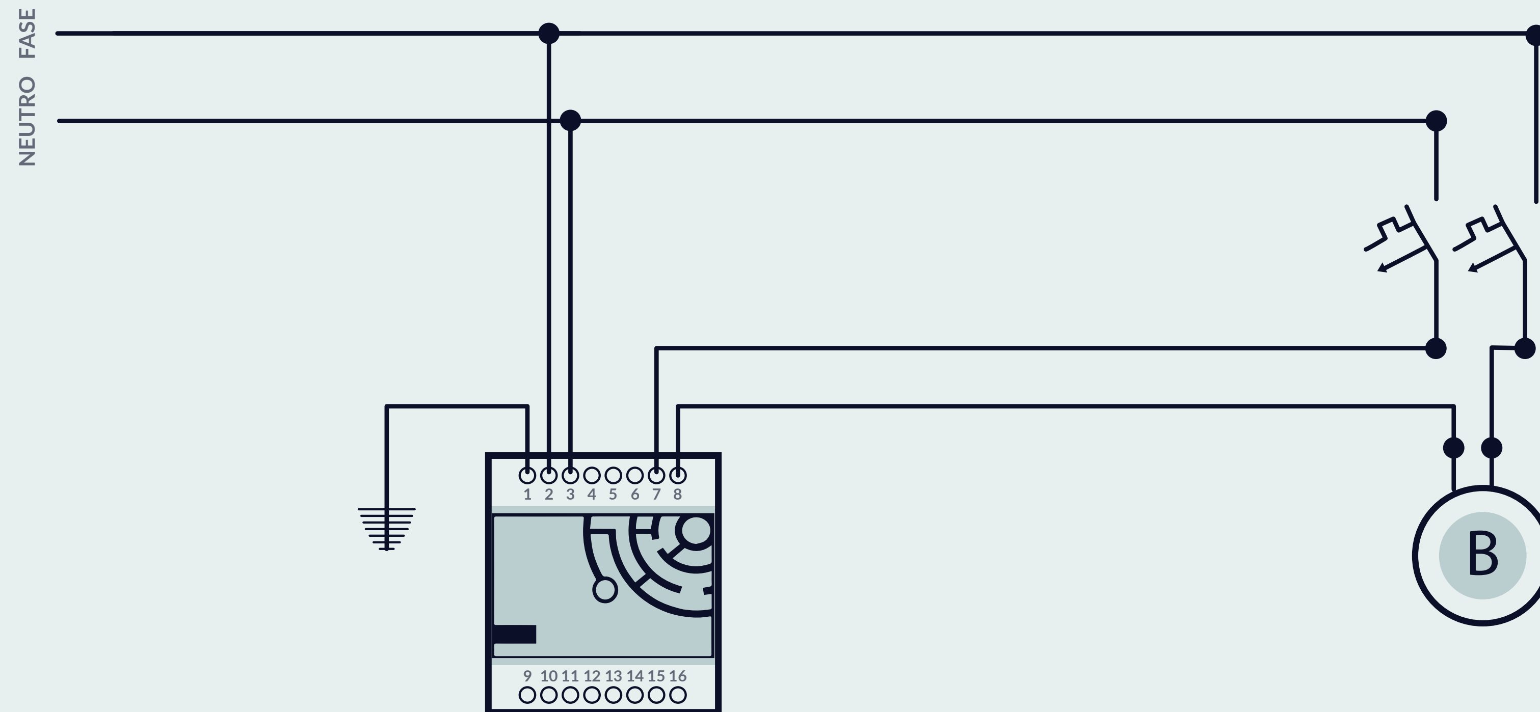
Figura 1: Esquema unifilar de conexión bomba monofásica
